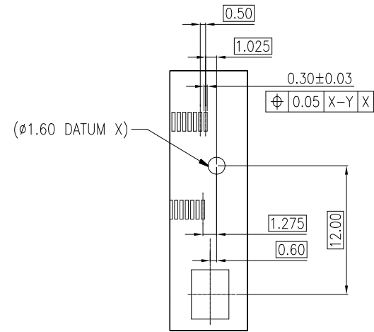
DETAIL:D SCALE 2:1
