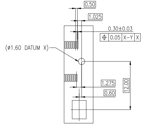
DETAIL:D SCALE 2:1
